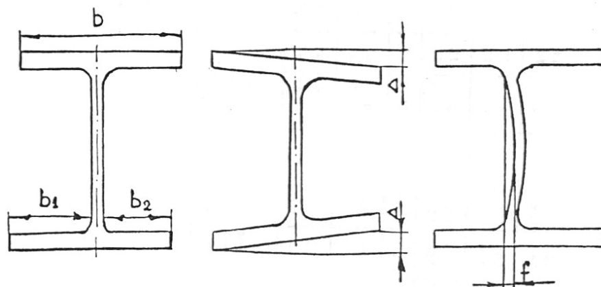
Чертеж 2
